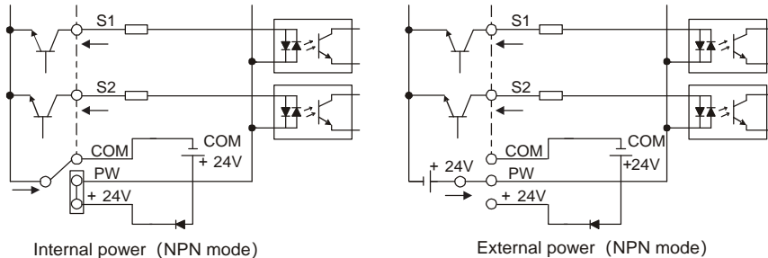
Рис 4.20 NPN режим
