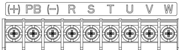
Рис 4.9 Клеммы силовых цепей 380 В 22 кВт и ниже
