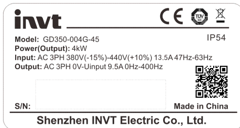
Рис 3.5 Табличка ПЧ
