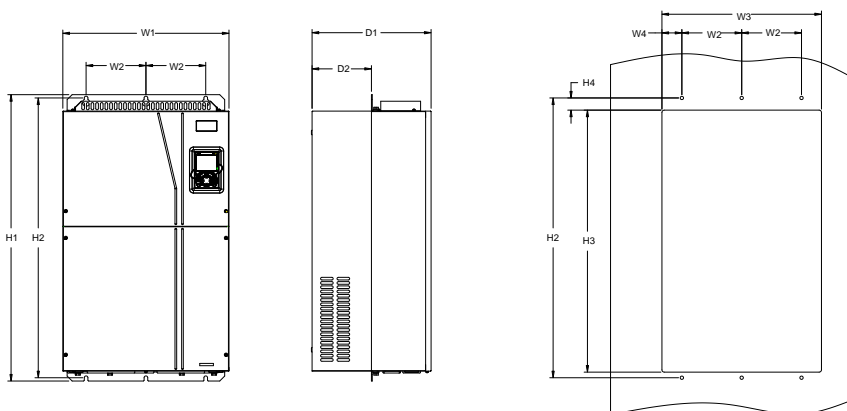
Рис 0.11 Схема фланцевого монтажа ПЧ напряжением 380 В, от 132 до 200 кВт
