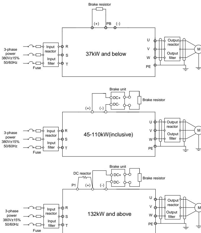
Рис 4.7 Схема подключения силовой цепи 380 В(-15%)–440 В(+10%)
